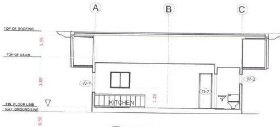
9 LONGITUDINAL SECTION A-9 SCALE 1:100 M
