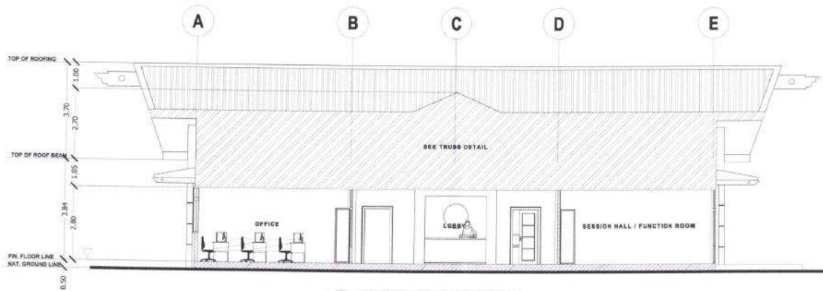
8 LONGITUDINAL SECTION A-B SCALE 1:100 M
